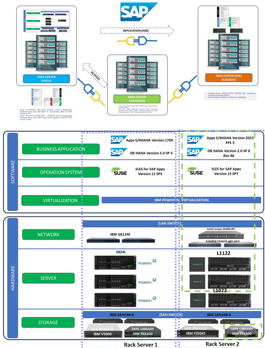
Gambar 1 Arsitektur Server ERP SAP
